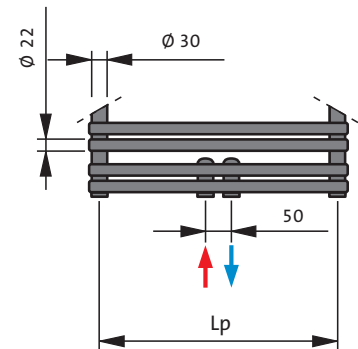
подсоединение
