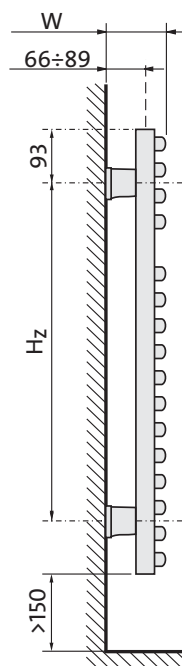
вид сбоку
