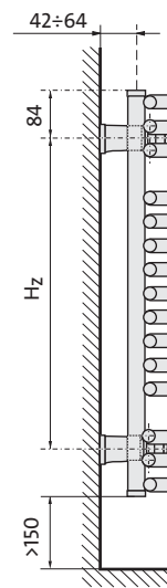
вид сбоку
