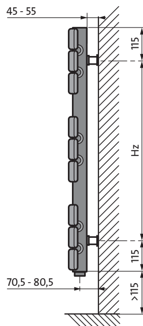
вид сбоку
