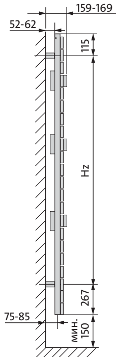
вид сбоку
