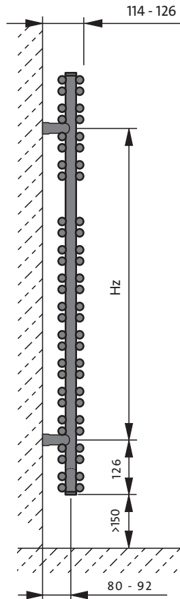
вид сбоку
