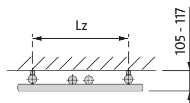
вид сверху
