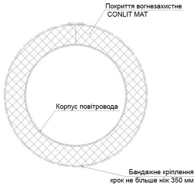
Мал. 1 а, б, в Монтаж системи за допомогою бандажного кріплення
