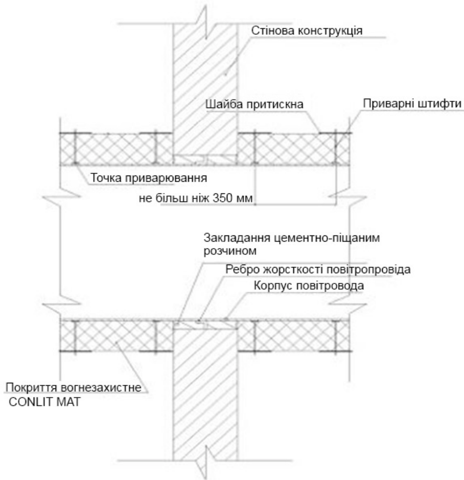
Мал. 5. Принципова схема перетину повітроводом будівельної конструкції
