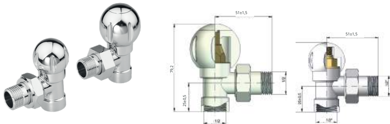
Регулювальний (ручний) комплект BALL, кутовий, ВР ½" / ЗР ½". Склад комплекту: регулювальний (ручний) кран BALL, зворотній клапан BALL.
